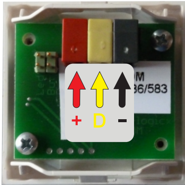
Aansluiting BDM
