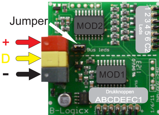
Aansluiting INM6K6L-24V
