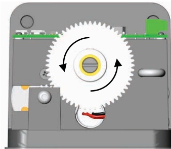
Door het grote tandwiel tegen de klok in te draaien, zal de pen naar buiten bewegen.
