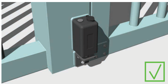
Slot neerwaarts verticaal gemonteerd op het frame van de poort
