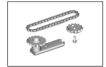
LT301 Arm tot 360°, opening met ketting.
