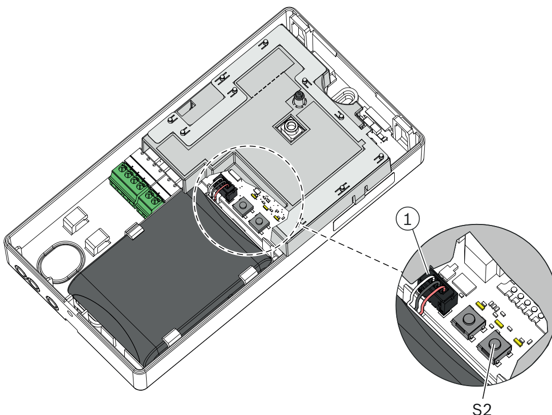
Afbeelding 7.1: Radiogateway FWI-270
