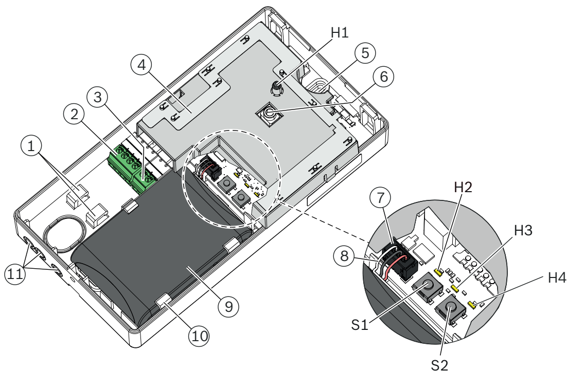
Afbeelding 3.3: Binnenaanzicht vanFWI-270
