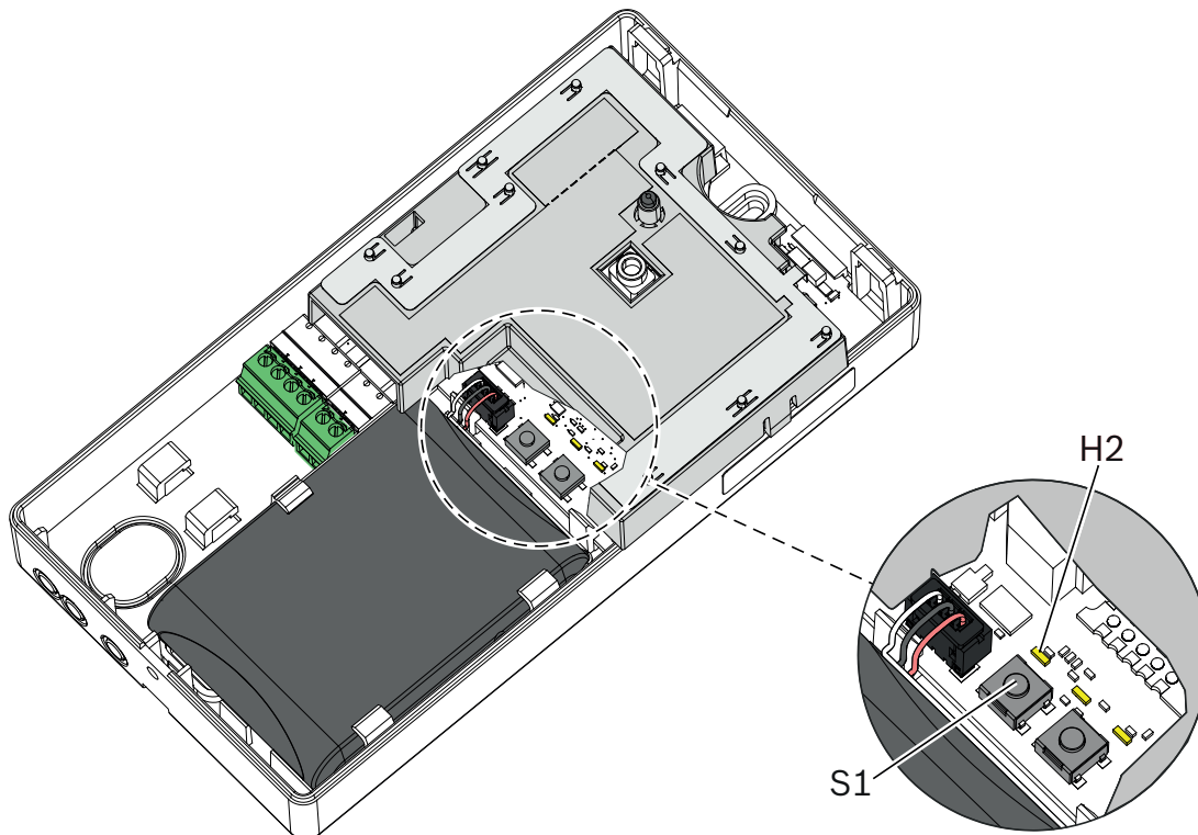
Afbeelding 7.3: Radiogateway FWI-270
