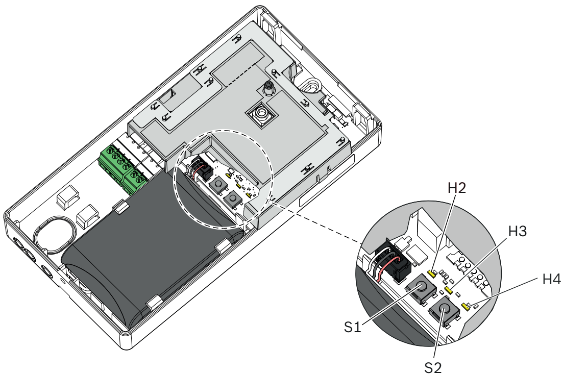
Afbeelding 7.5: Radiogateway FWI-270
