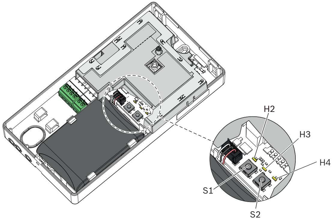
Afbeelding 7.4: Radiogateway FWI-270
