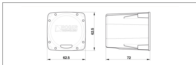
AFMETINGEN INGEBOUWDE DOOS
