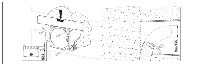
OPSTELLING VOOR STANDAARD INSTALLATIE INGEBOUWDE DOOS
